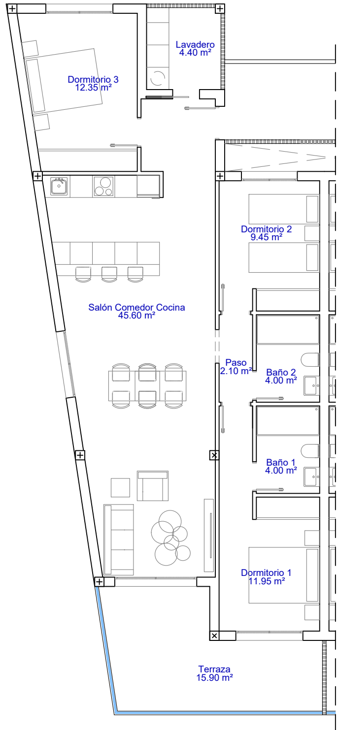
Planta Primera E:1/100
