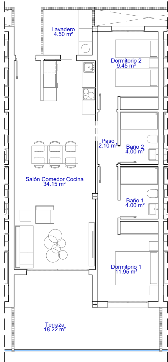
Planta Primera E:1/100
