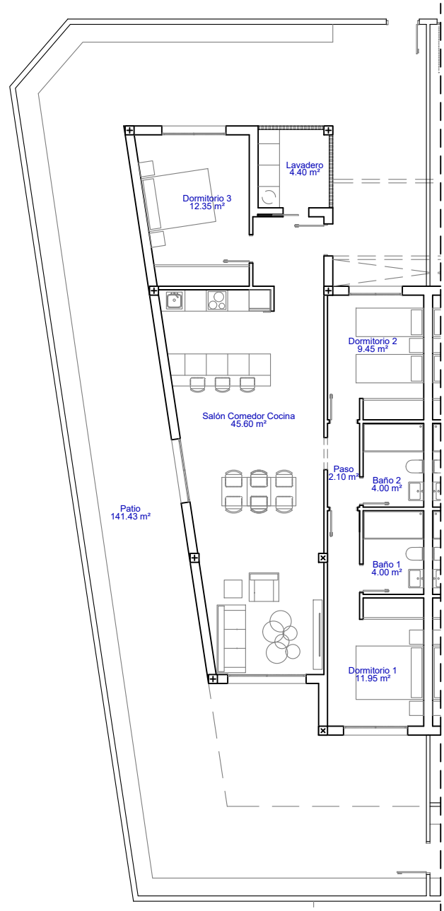
Planta Baja E:1/150
