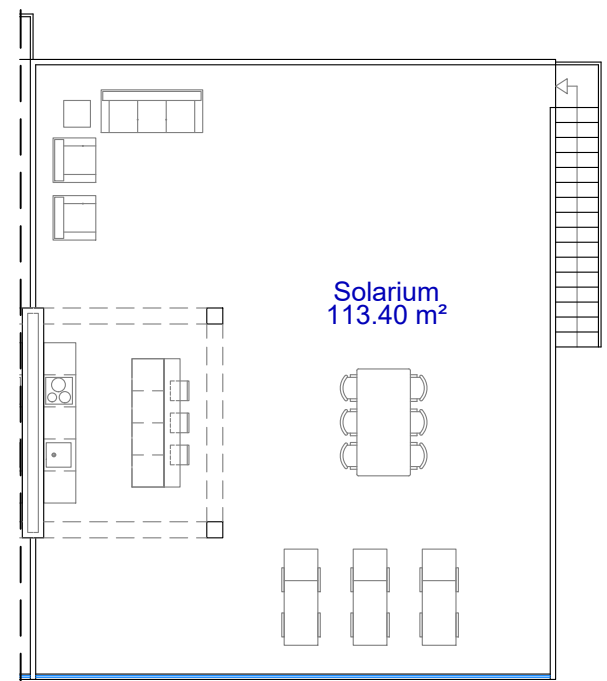
Planta Solarium E:1/200
