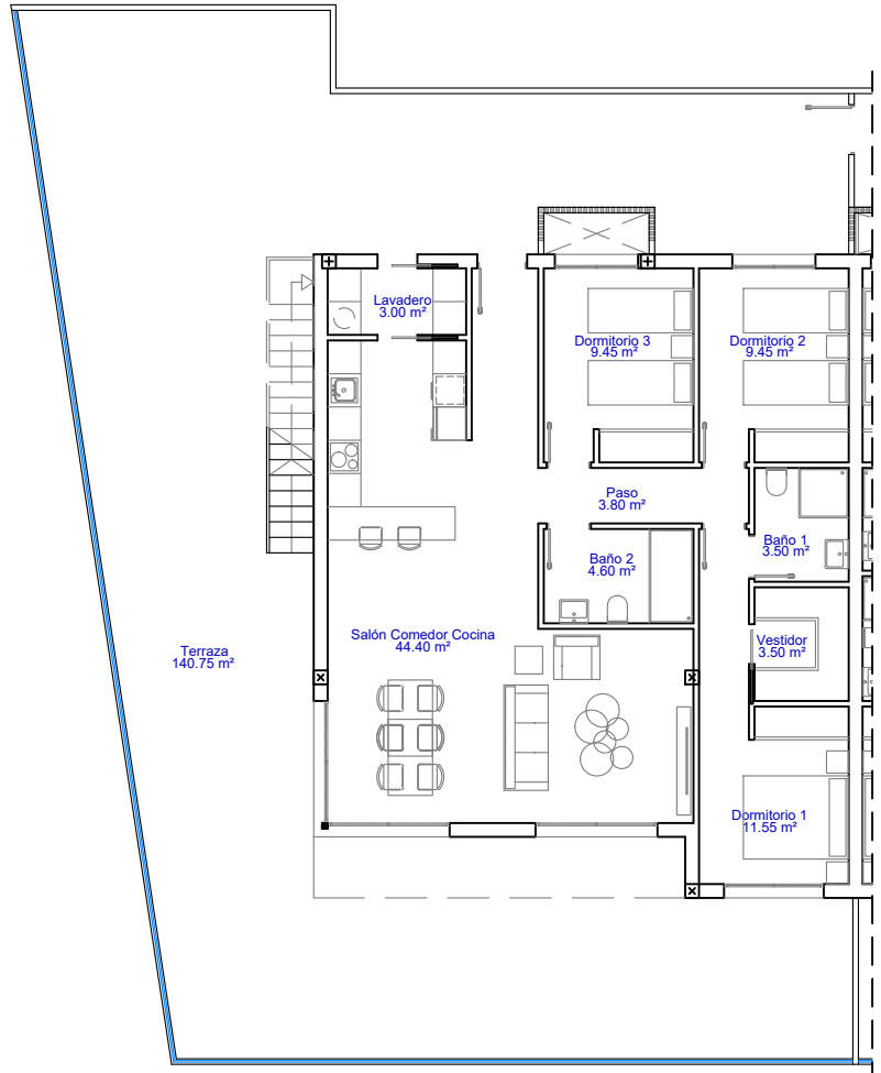
Planta Segunda E:1/150
