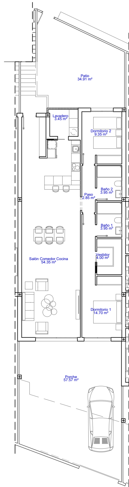
Planta Baja E:1/150
