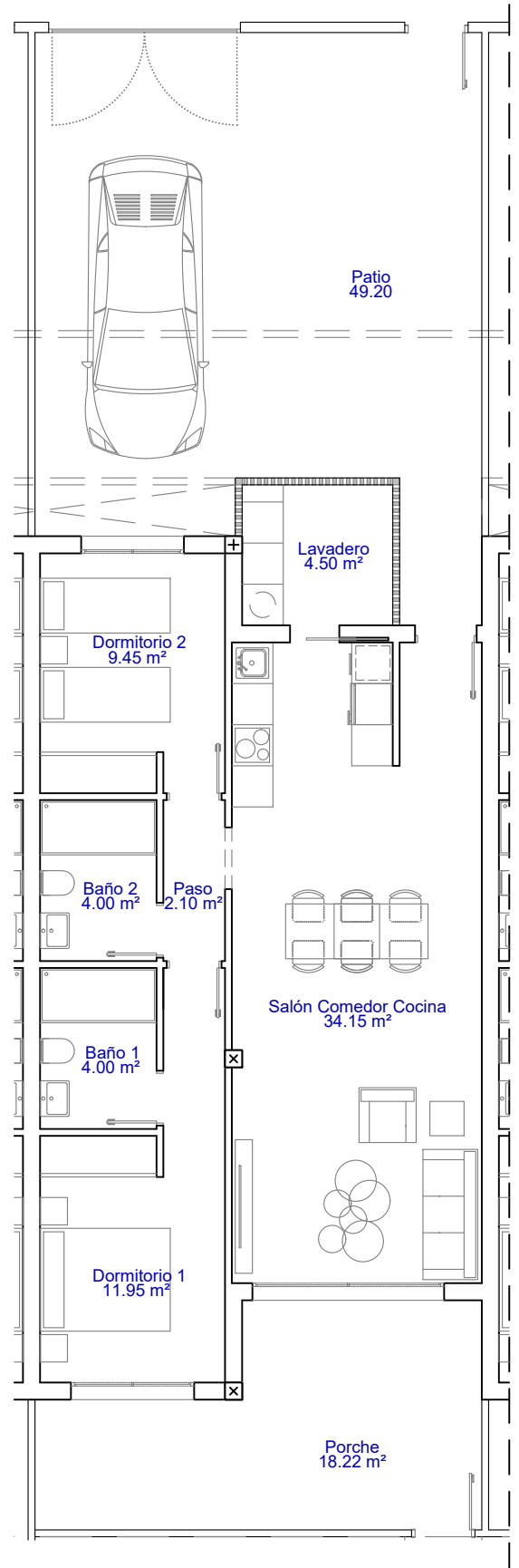
Planta Baja E:1/100
