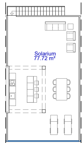
Planta Solarium E:1/200
